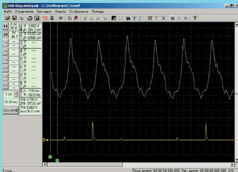
Сигнал синего цвета - разрежение во впускном коллекторе на работающем двигателе. Сигнал жёлтого цвета - импульс синхронизации от датчика синхронизации установленного на высоковольтный провод первого цилиндра. Порядок работы цилиндров - 1-3-4-2.
