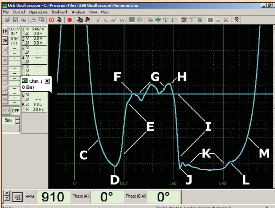
Тот же график, но с увеличенным усилением для лучшей наглядности участков выпуска отработавших газов и всасывания рабочей смеси.
