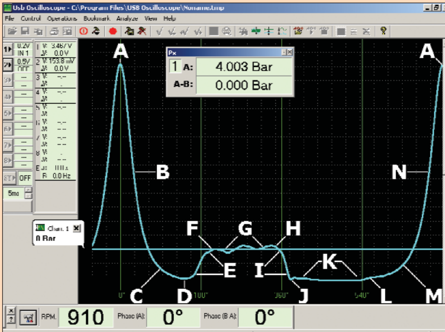
График давления в цилиндре и его характерные точки и участки прогретого до рабочей температуры исправного четырёхтактного четырёхцилиндрового бензинового двигателя, работающего на холостом ходу.
