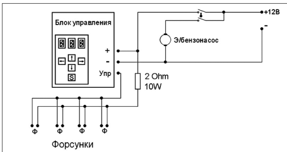
Рис. 11. Принципиальная электрическая схема стенда
