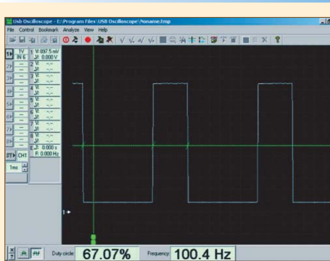
Рисунок 16. Осциллограмма напряжения сигнала управления клапаном холостого хода.
