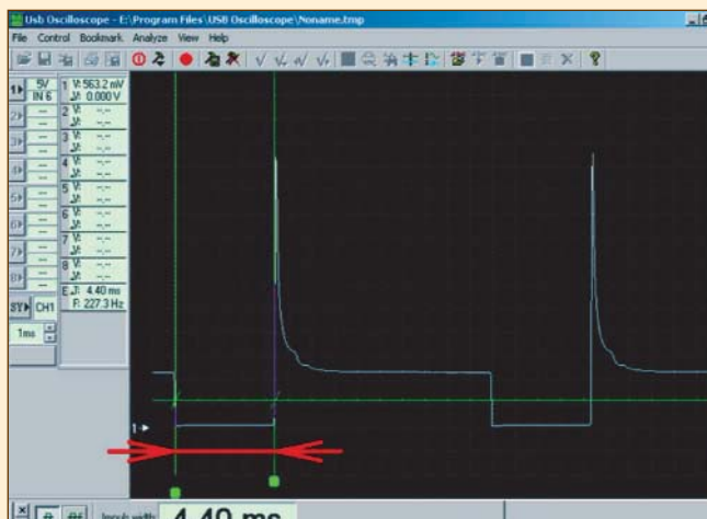
Рисунок 15. Осциллограмма напряжения сигнала управления. Impuls width: - длительность импульса.
