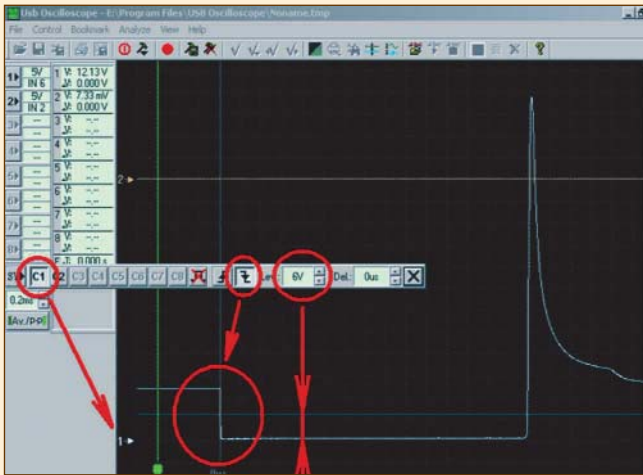
Рисунок 9. Пример настройки синхронизации. В данном случае синхронизация выбрана по заднему фронту сигнала канала №1 по уровню +6 Вольт.
