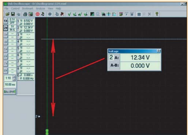
Рисунок 3. Осциллограмма напряжения автомобильной аккумуляторной батареи. А: - значение напряжения в момент времени указанный маркером. В данном случае соответствует напряжению автомобильной аккумуляторной батареи и равно ~12,3 Вольт.
