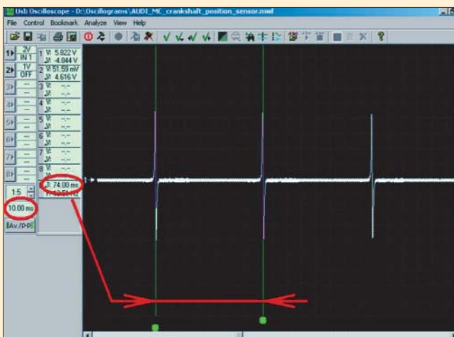
Рисунок 13. Осциллограмма выходного напряжения датчика положения коленчатого вала.
