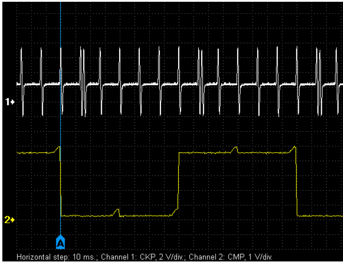
opel_astra_f_1993_1.4_c14nz.mwf
